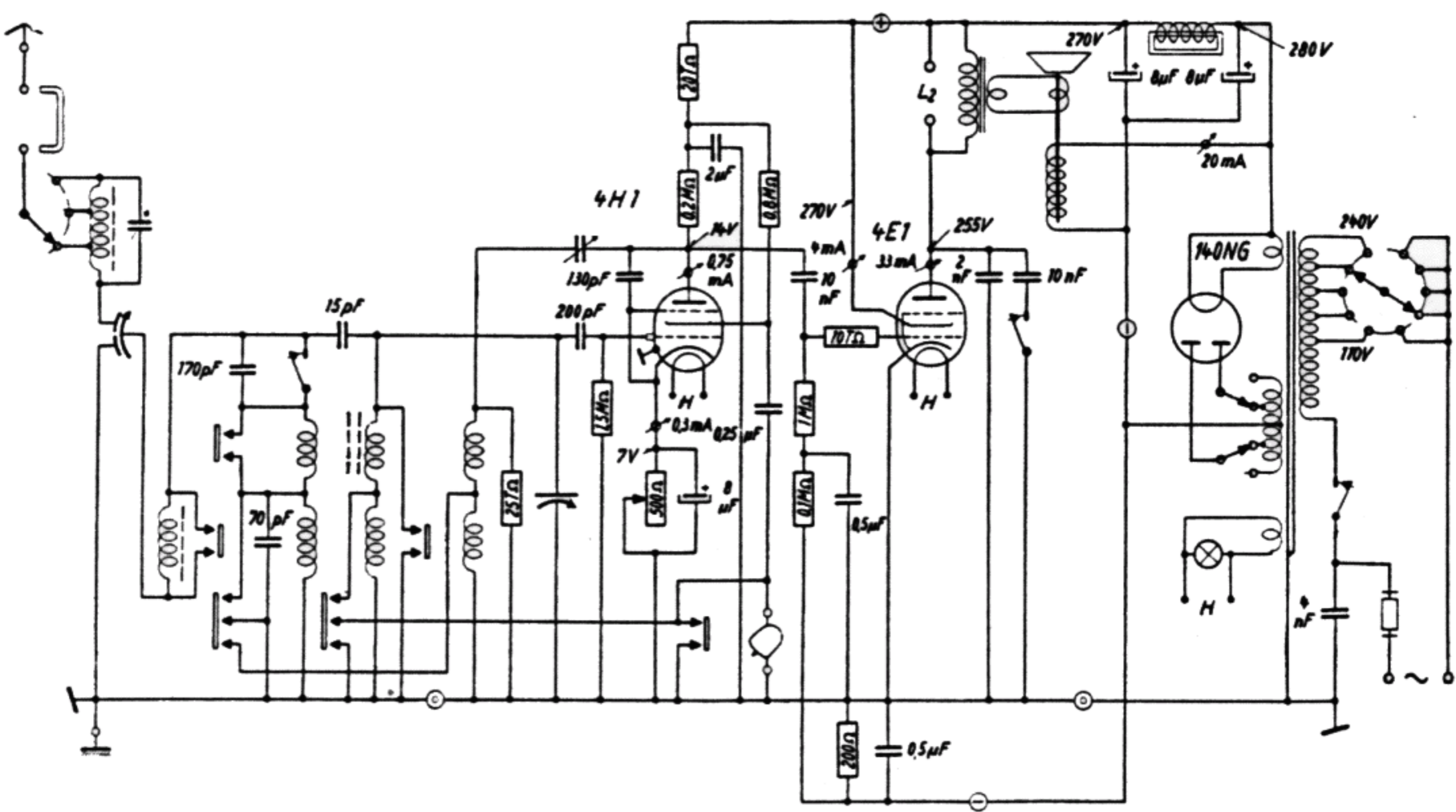
Loewe, Opta 138W, Wechselstrom, 1 Kreis
